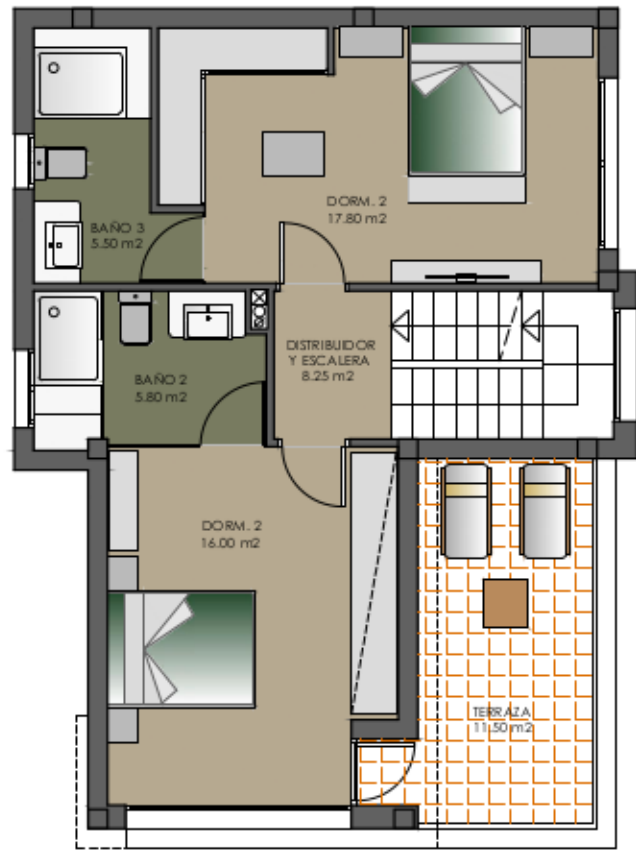
PLANTA PISO
