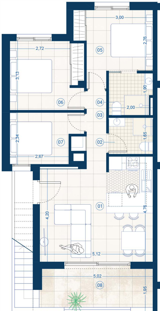
VIVIENDA EN PLANTA PRIMERA/HOUSE IN FIRST FLOOR
