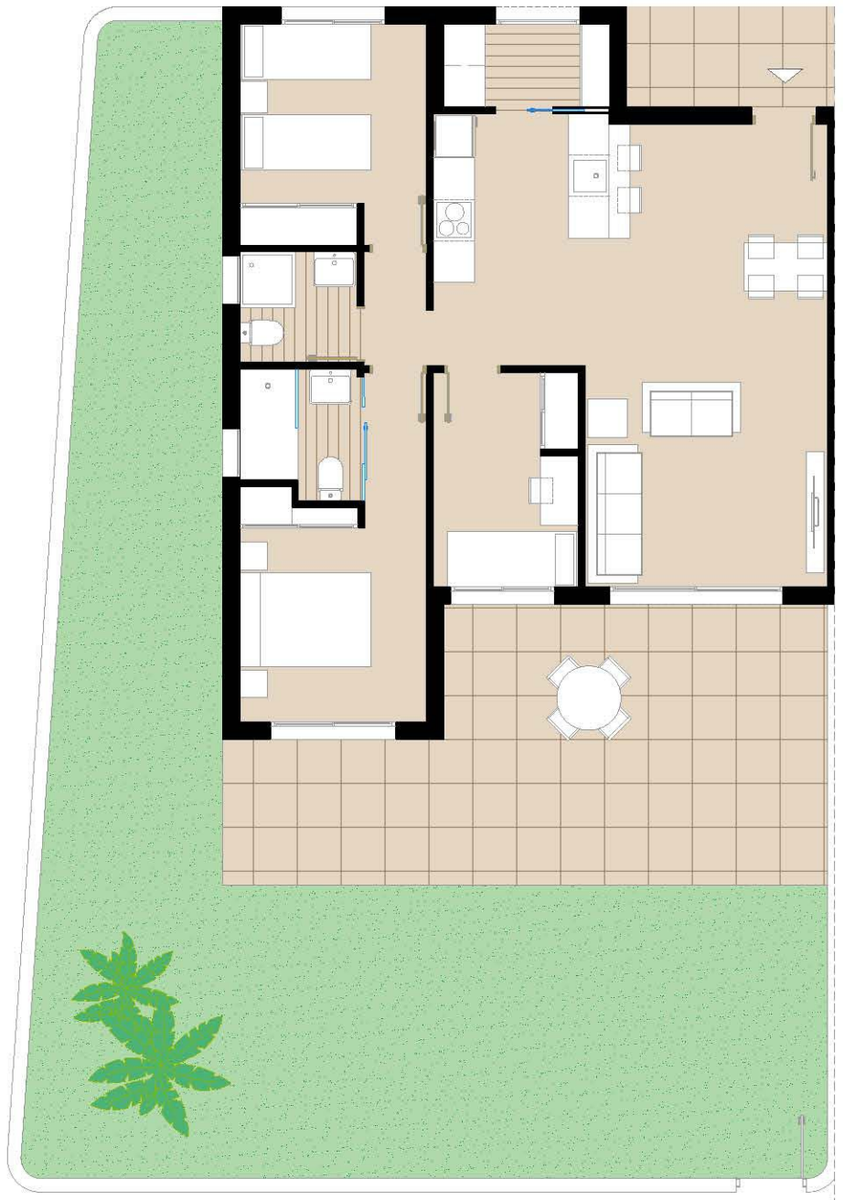
First Floor/ Planta Primera (E:1/100)
